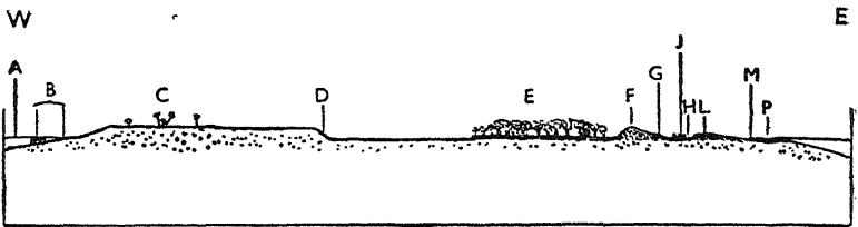
चित्र ९६ (a)—क्वीनलैंड के ग्रेट बेरियर रीफ के साथ छोटे वृक्षों वाले द्वीप (द्वीप शैलमाला) की अनुमानतः आकृति।
